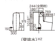
(壁排水) ※2
