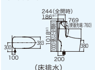
(床排水)
