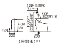
(床排水) ※1
