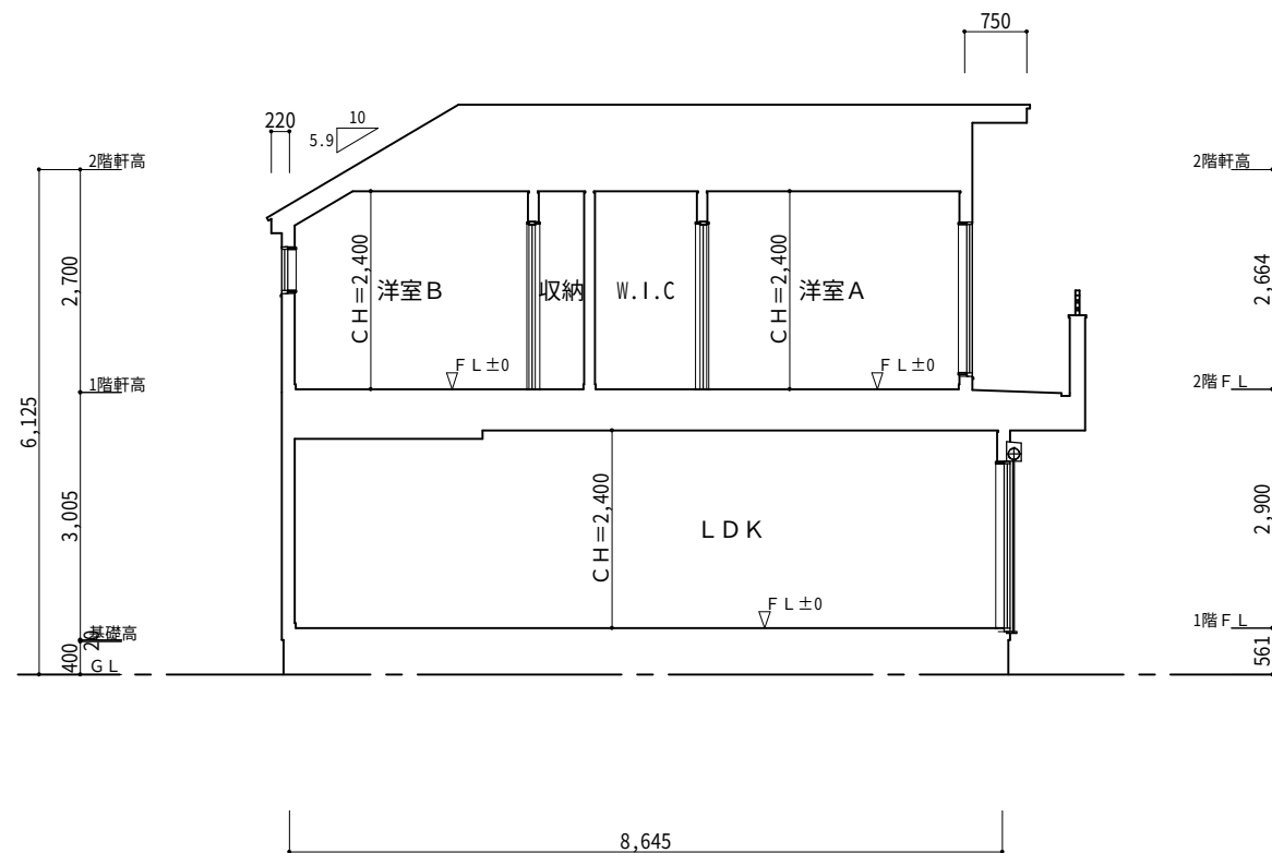
2面 断面図 S:1/100
