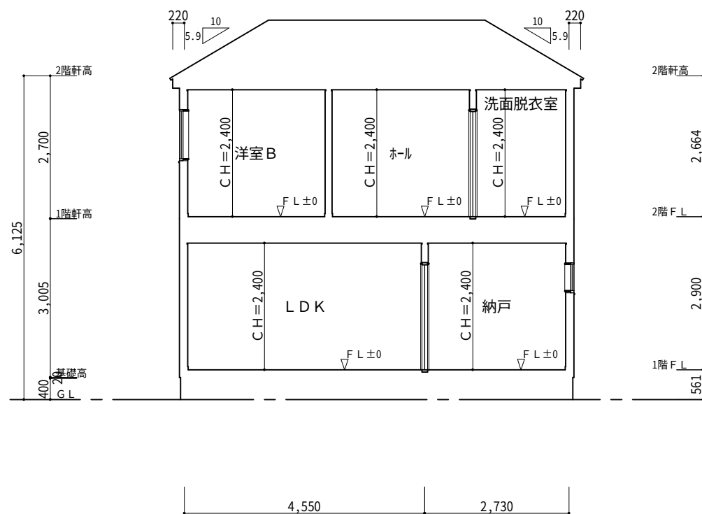
1面 断面図 S:1/100
