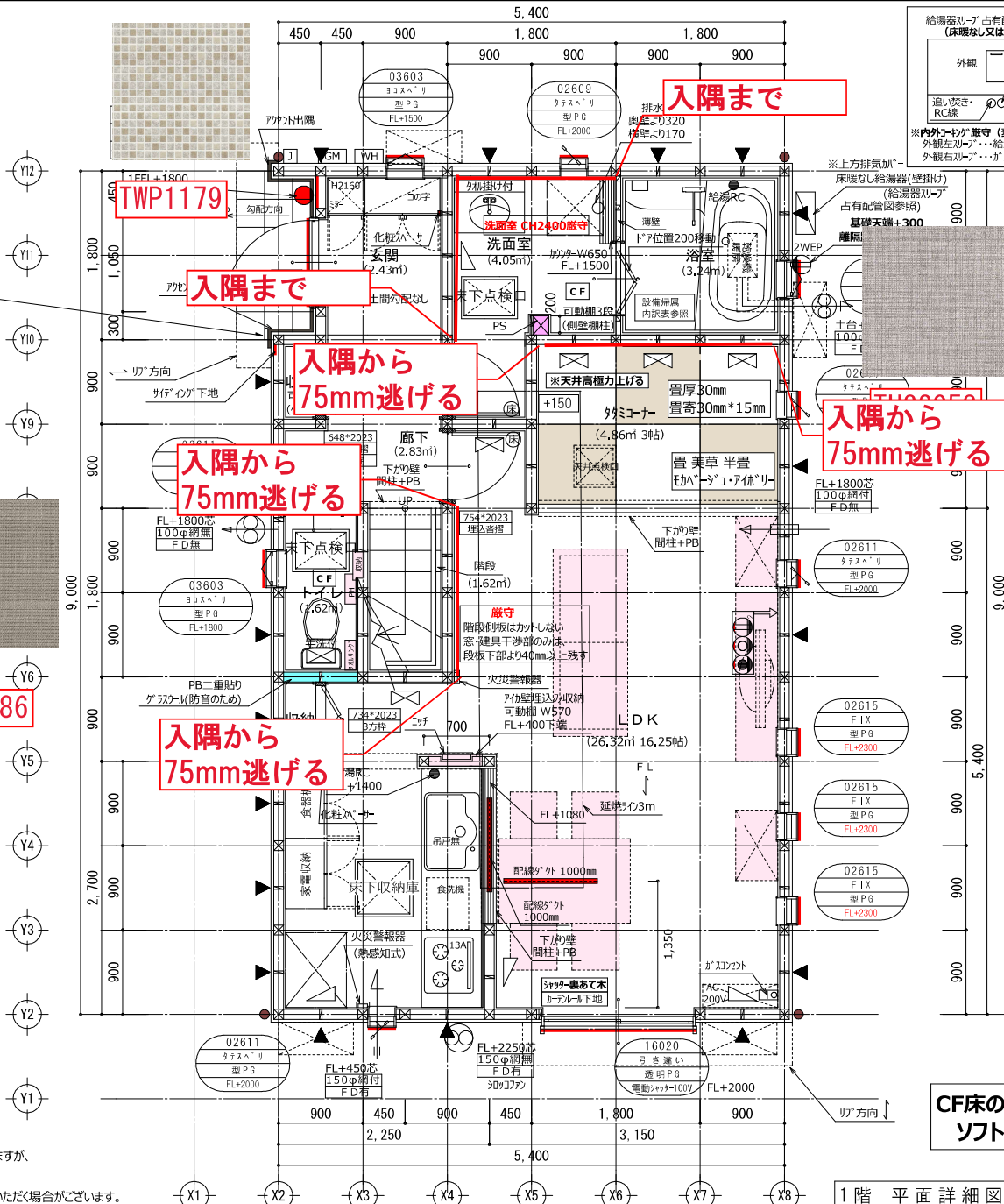
1階 平面詳細図 S:1/50
